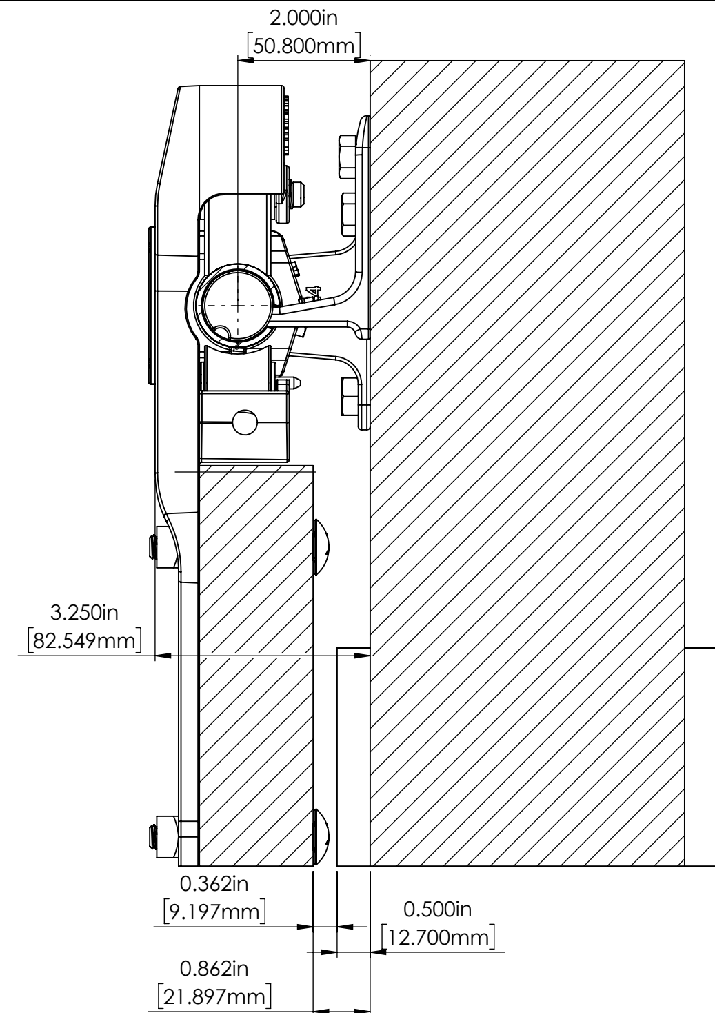
SECTION D-D SCALE 1 : 2
