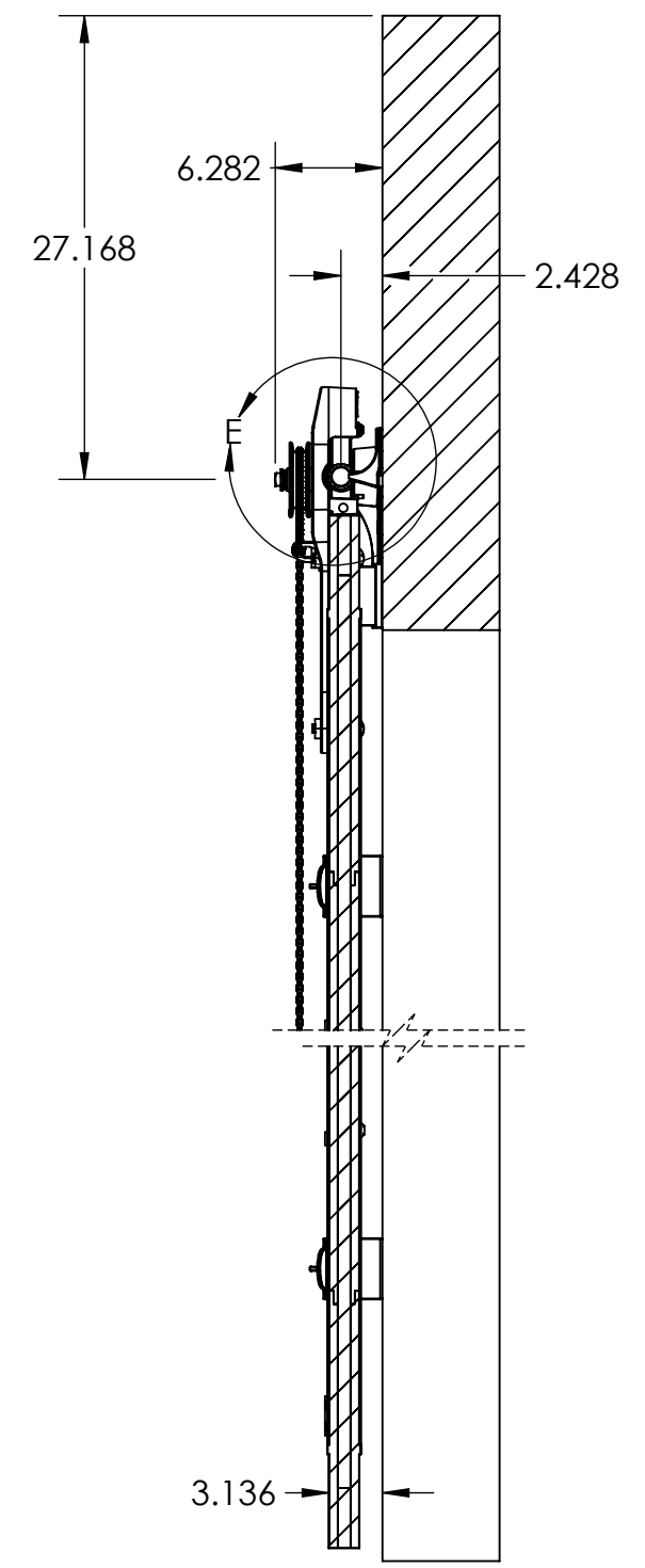
SECTION D-D SCALE 1 : 12
